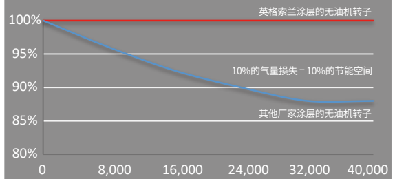
气量的变化: 英格索兰涂层vs 其他厂家涂层
